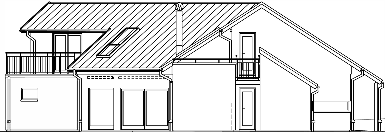
FASAD MOT ÖSTER
